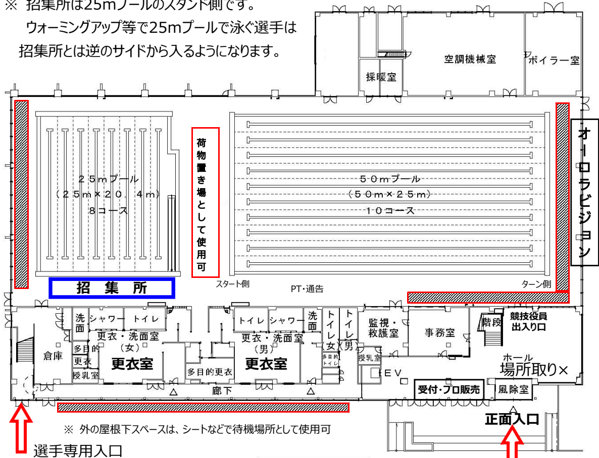
1階平面図
